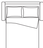
Divano letto da 210 L. 210 P. 101 H. 79/95 materasso 140x200 H. 12
